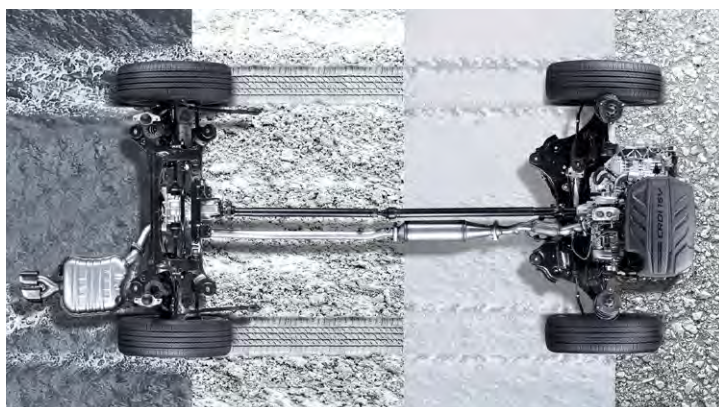
Układ napędu na cztery koła HTRAC™
